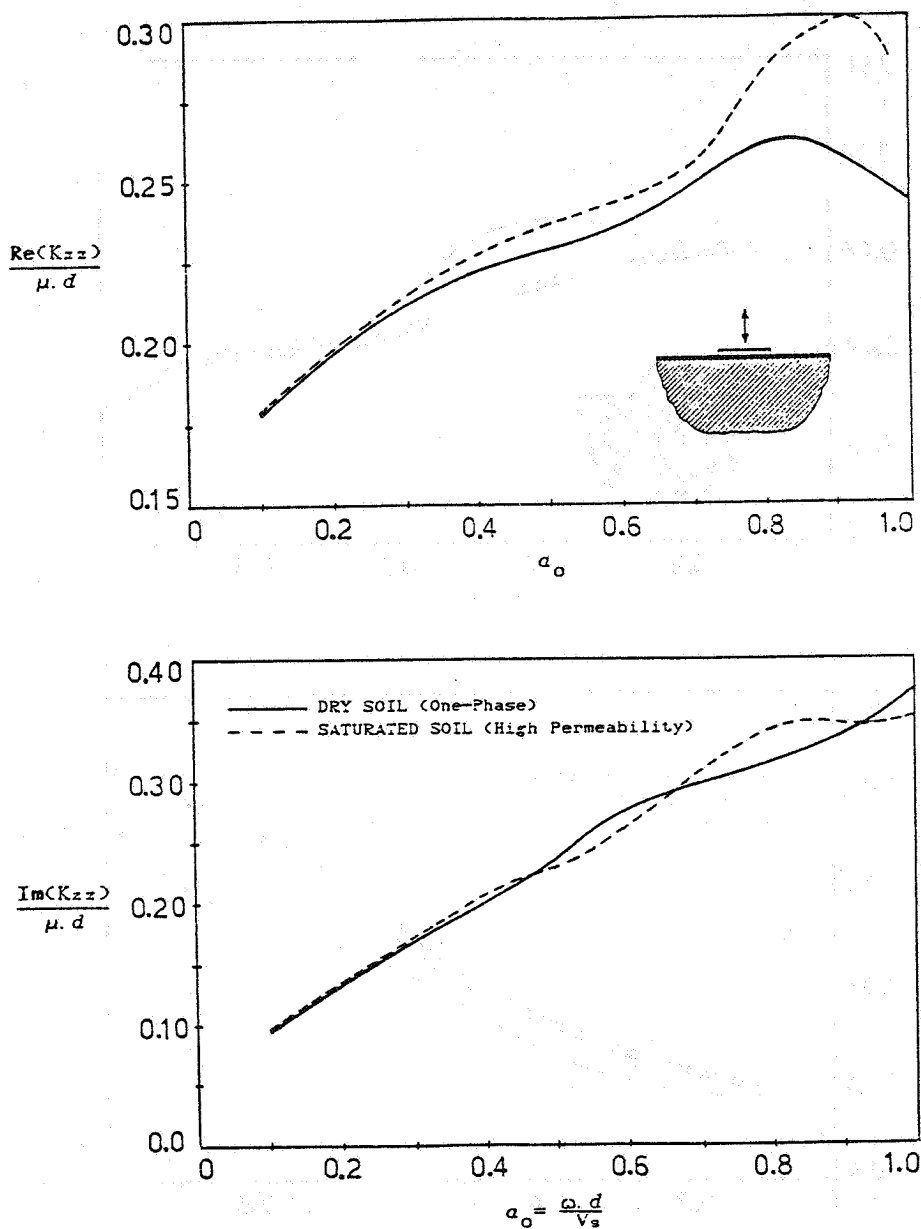
شکل ۹ - مقایسه محیط متخلخل اشباع با نفوذ پذیری بالا و محیط خشک تک فاز در تعیین سختی دینامیکی قائم پی صلب
