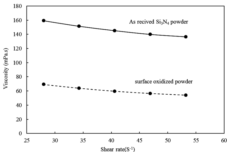
شکل ۴- تأثیر درصد پراکنده‌ساز بر گرانروی دوغاب نیتريد سيليسيم - نشاسته در نرخ برش ثابت ۵۰ بر ثانيه
