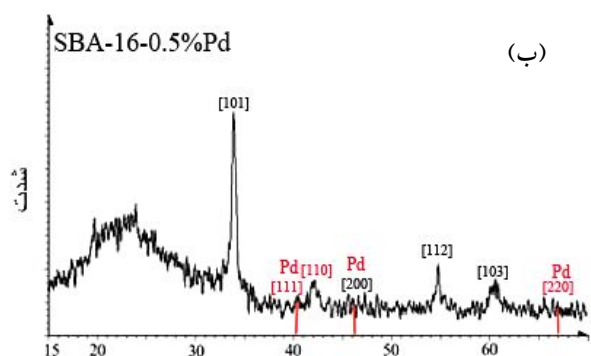
زاویه پراش بر حسب درجه (۲θ)
