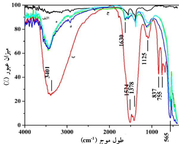
شکل ۷- طیف FT-IR الف) KBr خالص مورد استفاده، ب) رسوب حاصل و پودرهای کلسینه‌شده در دماهای ج) 900^{\circ}\text{C} د) 1000^{\circ}\text{C} و ه) 1100^{\circ}\text{C}
