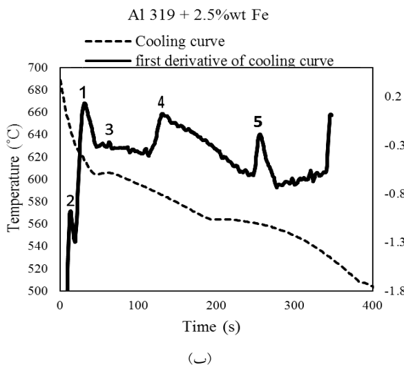
شکل ۴- نمودار سرد شدن و مشتق اول آن برای: الف) آلیاژ حاوی ۱/۵ درصد آهن و ب) آلیاژ حاوی ۲/۵ درصد آهن
