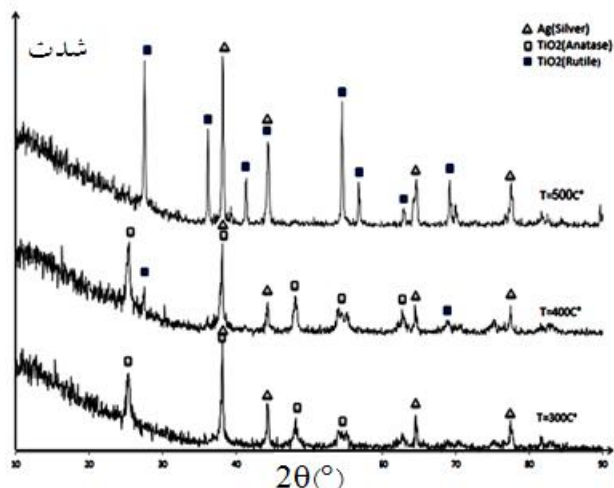
شکل ۱- الگوی پراش پرتو ایکس از نانوترکیب Ag-TiO_2 در دماهای مختلف
