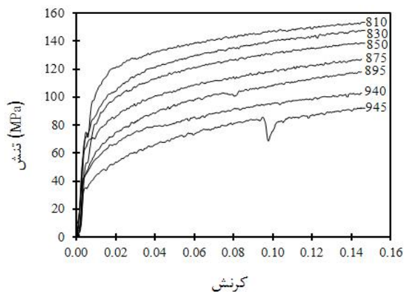
شکل ۲- منحنی‌های مربوط به تنش سیلان فولاد مورد پژوهش در دماهای مختلف (بر حسب درجه سانتی‌گراد)
