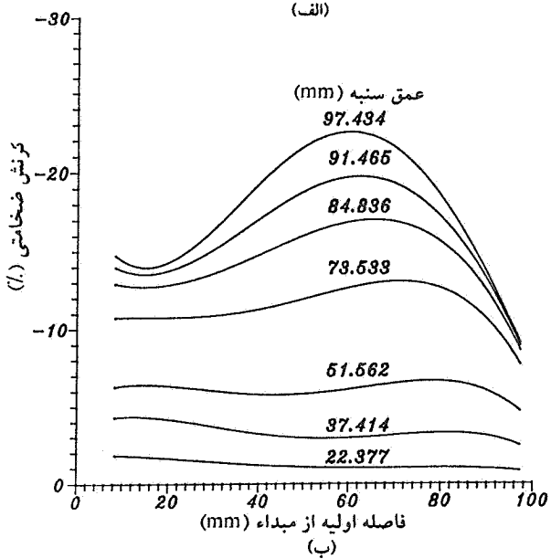
شکل ۷- منحنیهای توزیع کرنش در جهت ضخامت در کورسهای مختلف
