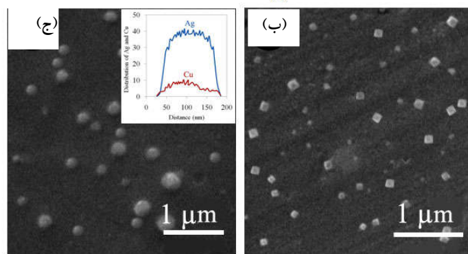
شکل ۳- الف) الگوی پراش پرتو ایکس در دو حالت حضور آمونیا و عدم حضور آمونیا در سنتز نانوذرات آلیاژی نقره- مس، ب) تصویر میکروسکوپی الکترونی روبشی نانوذرات نقره- اکسید مس و ج) تصویر میکروسکوپی الکترونی روبشی نانوذرات نقره- مس (تصویر درونی نشان‌دهنده آنالیز عنصری از یک نانوذره است)
