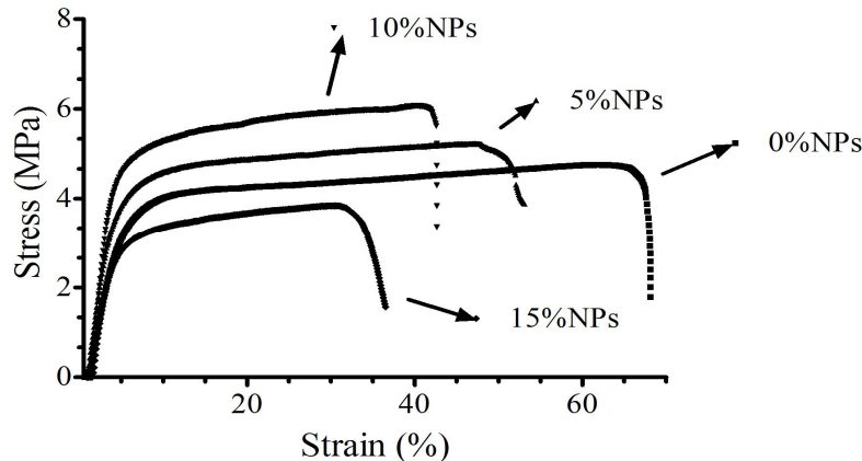
شکل ۲- نمودار تنش - کرنش نمونه داربست‌های نانولیفی حاوی مقادیر مختلف نانوذره HBR (NPs)
