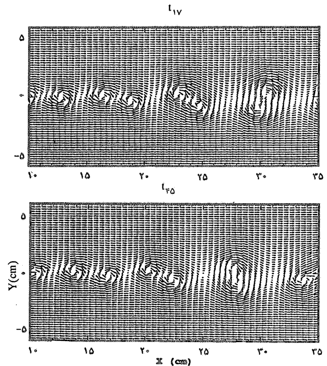
شکل ۶ - میدان بردارهای سرعت برای دو تصویر مرکب در t_{17} و t_{45}
