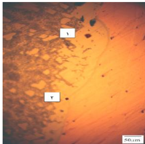
شکل ۹- اثرات فرورونده هرمی در آزمون ریزسختی سنجی در نمونه A800C25. نقطه ۱ واقع در منطقه فاز ۱ و نقطه ۲ واقع در منطقه ۲ است.
