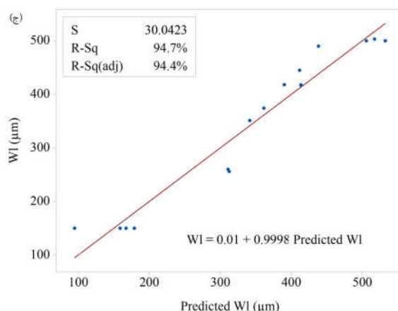
شکل ۳- نمودار پراکنندگی مقادیر اندازه‌گیری شده بر حسب مقادیر تخمینی برای مدل‌های: الف) عرض بالایی جوش، ب) عرض میانی جوش و ج) عرض پایینی جوش
