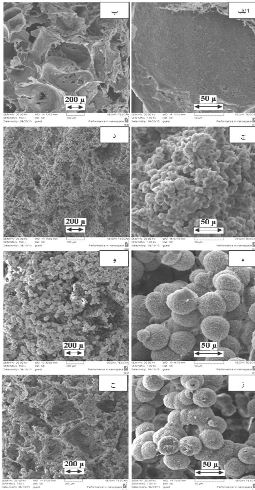
شکل ۲- تصاویر میکروسکوپی الکترونی روبشی از مورفولوژی مقطع عرضی الف) داربست ۱ با بزرگ‌نمایی 1k× ب) داربست ۱ با بزرگ‌نمایی 150× (ج) داربست 1 با بزرگ‌نمایی 1k× (د) داربست 1 تصویر با بزرگ‌نمایی 150× ه) داربست 2 با بزرگ‌نمایی 1k× (و) داربست 2 با بزرگ‌نمایی 150× (ز) داربست 3 با بزرگ‌نمایی 1k× (ح) داربست 3 با بزرگ‌نمایی 150×
