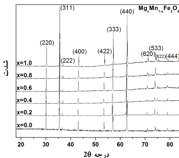
شکل ۳- الگوی پراش پرتو ایکس فریت Mg_xMn_{1-x}Fe_2O_4 در دمای تفجوشی ۱۲۵۰ درجه سانتی‌گراد
