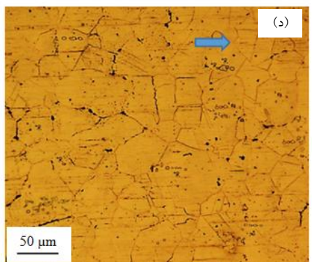
شکل ۱- ریزساختار Hastelloy X تحت عملیات حرارتی آیل در دمای ۱۱۷۵ درجه سانتی‌گراد: الف) فاقد منیزیم، ب) حاوی ۱۷ ppm، ج) حاوی ۳۳ ppm و د) حاوی ۴۷ ppm منیزیم
