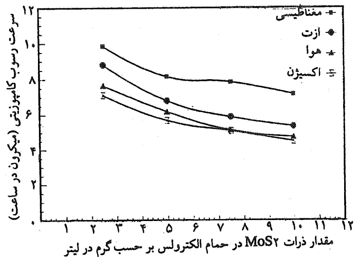
شکل ۲- تأثیر میزان بارگذاری ذرات MOS 2 در حمام روی سرعت رسوب میکرومتر یا از تغییرات وزنی به وسیله ترازوهای دقیق و از میکروسکوپ الکترونی روبشی و میکروسکپ نوری برای بررسیهای توپوگرافی و متالوگرافی استفاده شد. از به هم زدن مغناطیسی با گرم کننده الکتریکی و در شرایط به هم زدن با گاز از هوا، اکسیژن و ازت همراه با سیستم گرم کننده گاز استفاده شد. دمای گاز قبل از ورود به حمام حدود ۵۰ درجه سانتی گراد بود. برای تغییر در سرعت دمیدن گاز نیز از سیستم کنترل فلومتر استفاده شد.
