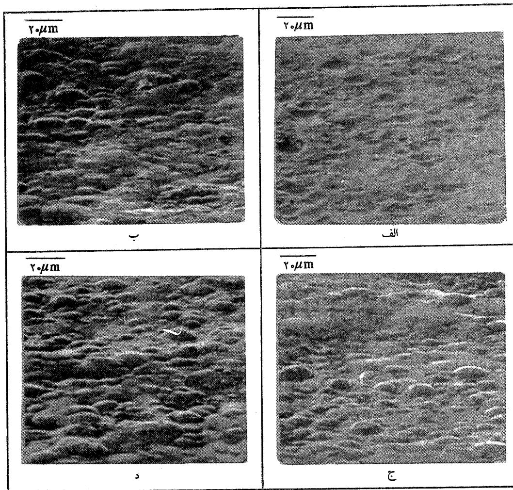
شکل ۹- تصاویر SEM پوشش کامپوزیتی الکتروپلوس Ni-P-MoS_3 تحت سرعت‌های مختلف دمیدن اکسیژن در حمام، زمان آبکاری ۴ ساعت
