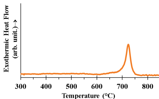
شکل ۸- منحنی گرماسنجی روبشی تفاضلی آلیاژ آمورف Ni_{55}Nb_{35}Si_{10} با نرخ گرم شدن 10^\circ درجه سانتی‌گراد بر دقیقه
