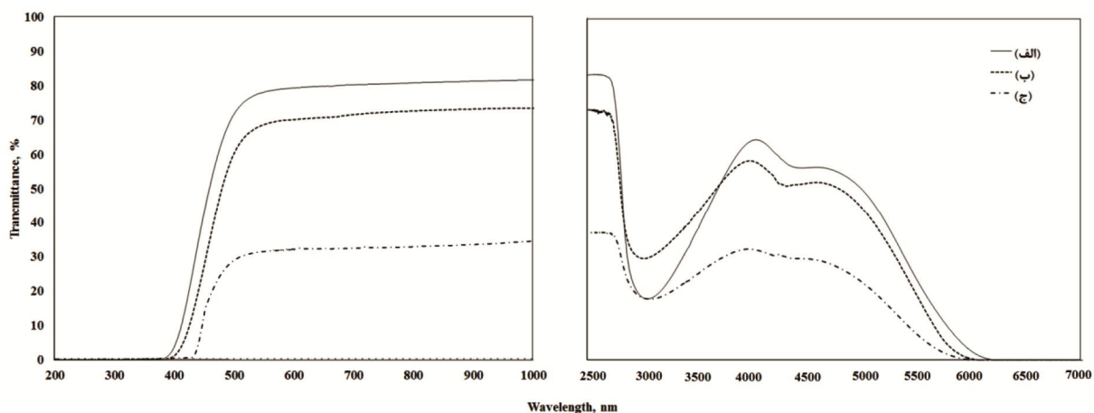
شکل ۶- نمودارهای عبورپذیری مربوط به شیشه‌های 50\text{GeO}_2-(50-x)\text{PbO}-x\text{CaO} در حضور: (الف) صفر، (ب) 10^\circ و (ج) 20^\circ درصد مولی اکسید کلسیم (با ضخامت سه میلی‌متر)
