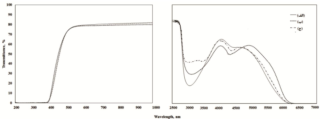
شکل ۷- نمودارهای عبورپذیری مربوط به شیشه‌های 50\text{GeO}_2-(50-x)\text{PbO}-x\text{SrO} در حضور: (الف) صفر، (ب) 10^\circ و (ج) 20^\circ درصد مولی اکسید استرانسیم (با ضخامت سه میلی‌متر)
