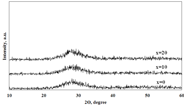
شکل ۲- الگوهای پراش پرتو ایکس مربوط به شیشه‌های 5\text{-}x\text{PbO-xSrO-GeO}_2 در حضور صفر، ۱۰ و ۲۰ درصد مولی اکسید کلسیم
