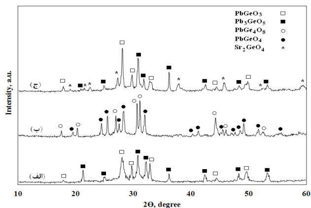
شکل ۵- الگوهای پراش پرتو ایکس نمونه‌های: (الف) 50\text{GeO}_2-50\text{PbO} ، (ب) 50\text{GeO}_2-40\text{PbO}-10\text{CaO} و (ج) 50\text{GeO}_2-40\text{PbO}-10\text{SrO} پس از انجام عملیات حرارتی در دمای 850^\circ\text{C} درجه سانتی‌گراد به مدت یک ساعت
