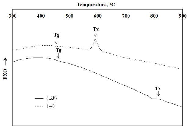
شکل ۳- نمودارهای آنالیز حرارتی مربوط به شیشه‌های 5\text{-}x\text{PbO-xCaO-GeO}_2 در حضور: الف) صفر و ب) ۱۰ درصد مولی اکسید کلسیم
