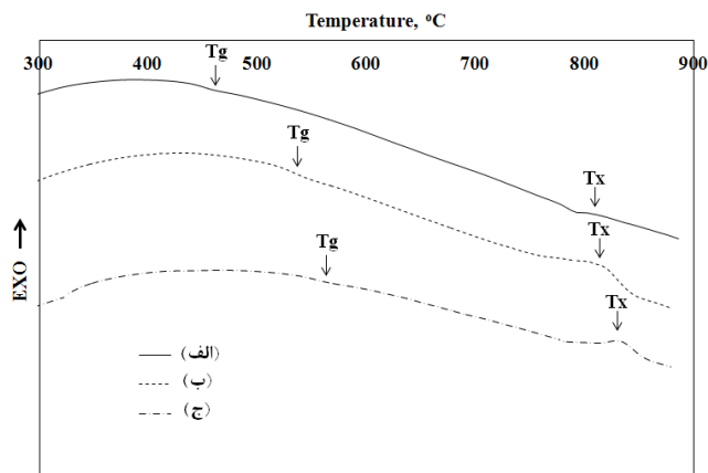
شکل ۴- نمودارهای آنالیز حرارتی مربوط به شیشه‌های 5\text{-}x\text{PbO-xSrO-GeO}_2 در حضور: الف) صفر، ب) ۱۰ و ج) ۲۰ درصد مولی اکسید استرانسیم
