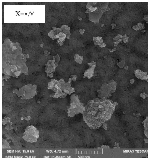
شکل ۳- تصاویر میکروسکوپی الکترونی روبشی نمونه‌های فریت کبالت آرایش یافته با کروم به‌ازای درصدهای مختلف آرایش
