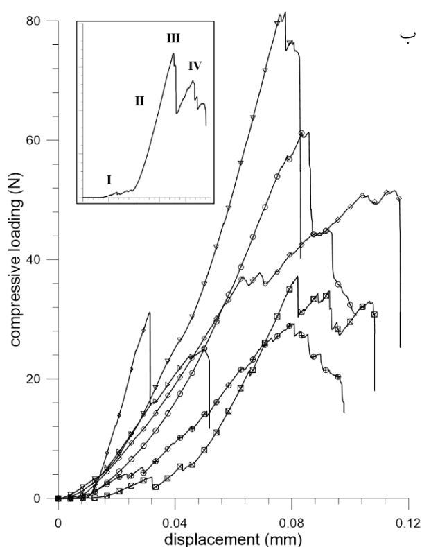
شکل ۳- الف) منحنی های نیروی فشاری - جابه جایی برای پایه های ماکرومخلخل در اندازه حفره های مختلف، ب) بزرگنمایی قسمت مشخص شده در تصویر الف (نواحی مختلف منحنی برای نمونه RPC80_C3 در گوشه بالایی سمت چپ این تصویر شماره گذاری شده اند.)
