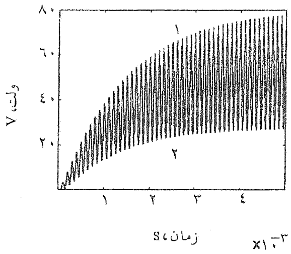
شکل ۶ - مبدل معکوس کننده ولتاژ و ولتاژ (۱) منحنی واقعی و (۲) تقریب مرتبه اول
