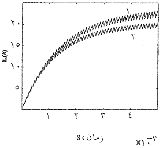
شکل ۶ - مبدل معکوس کننده ولتاژ و ولتاژ (۱) منحنی واقعی و (۲) تقریب مرتبه اول
