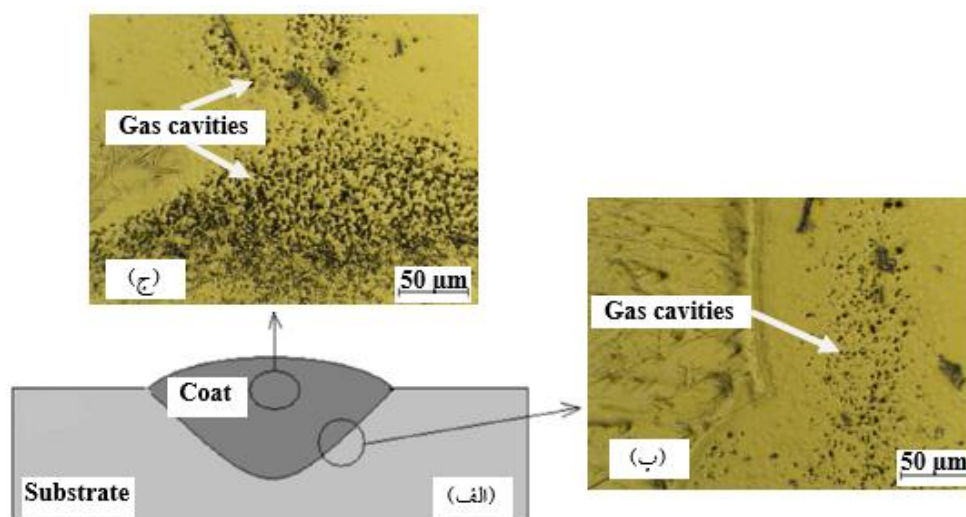
شکل ۱۹- الف) طرحواره‌ای از پوشش و زیرلایه تیتانیوم، ب) تصویر میکروسکوپی نوری از عیوب اطراف خط ذوب و ج) تصویر میکروسکوپی نوری از عیوب موجود در خط مرکزی جوش
