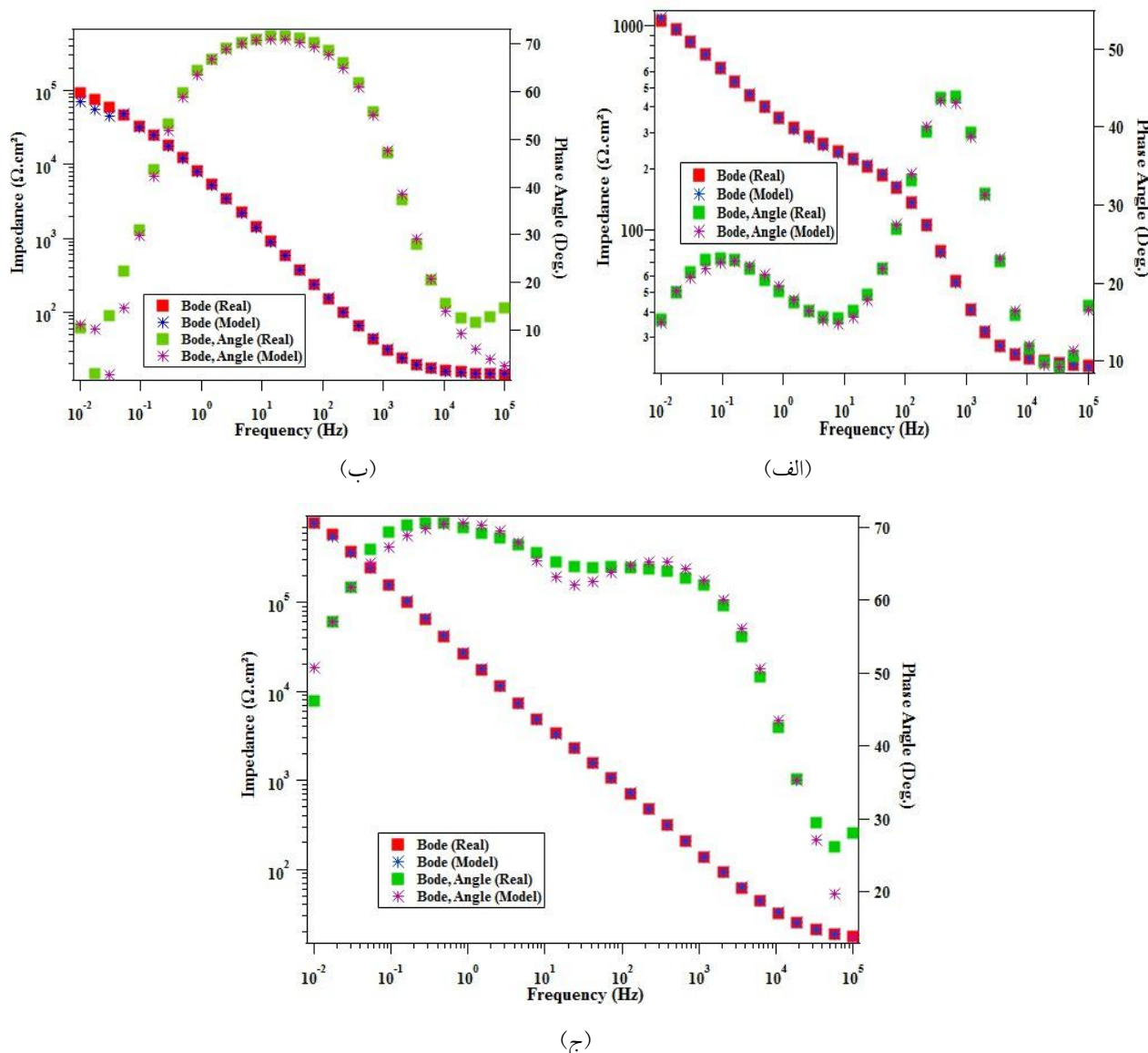
شکل ۱۸- نتایج انطباق نقاط به دست آمده از آزمون (منحنی‌های بد و بد- فاز) (Real) با نقاط حاصل از شبیه‌سازی توسط مدار الکتریکی (Model): الف) نمونه ۱، ب) نمونه ۲ و ج) نمونه ۳
