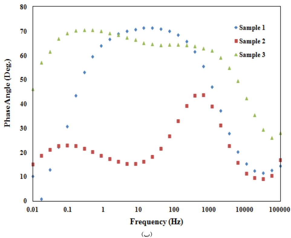
شکل ۱۷- الف) منحنی‌های بد (امپدانس نسبت به فرکانس) و ب) منحنی‌های بد- فاز (زاویه فاز نسبت به فرکانس) برای نمونه‌های تیتانیم خالص (Sample 1)، تهیه شده در اتمسفر آرگون (Sample 2) و تهیه شده در اتمسفر آرگون حاوی نیتروژن (Sample 3) در محلول ۳/۵ درصد سدیم کلرید
