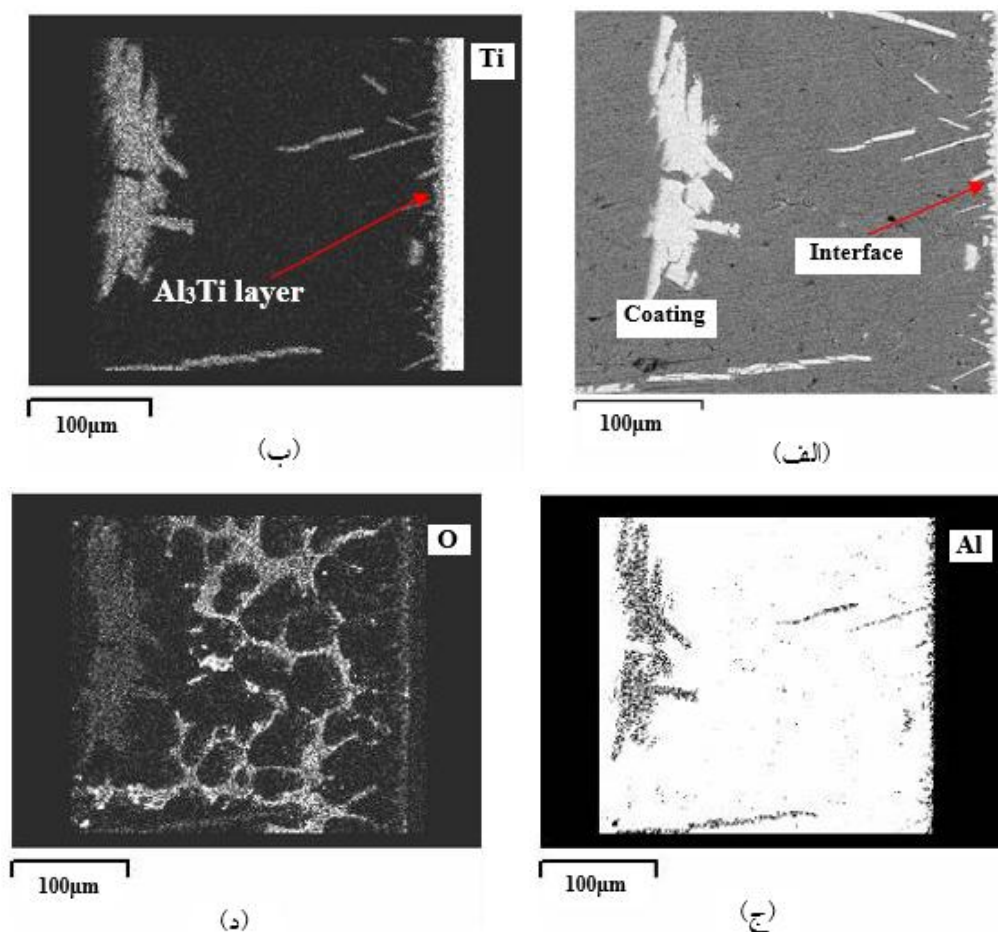
شکل ۷- الف) تصویر میکروسکوپی الکترونی روبشی از نمونه کامپوزیتی حاصل در حضور گاز محافظ آرگون خالص، ب) نقشه توزیع عنصر تیتانیوم، ج) نقشه توزیع عنصر آلومینیم و د) نقشه توزیع عنصر اکسیژن
