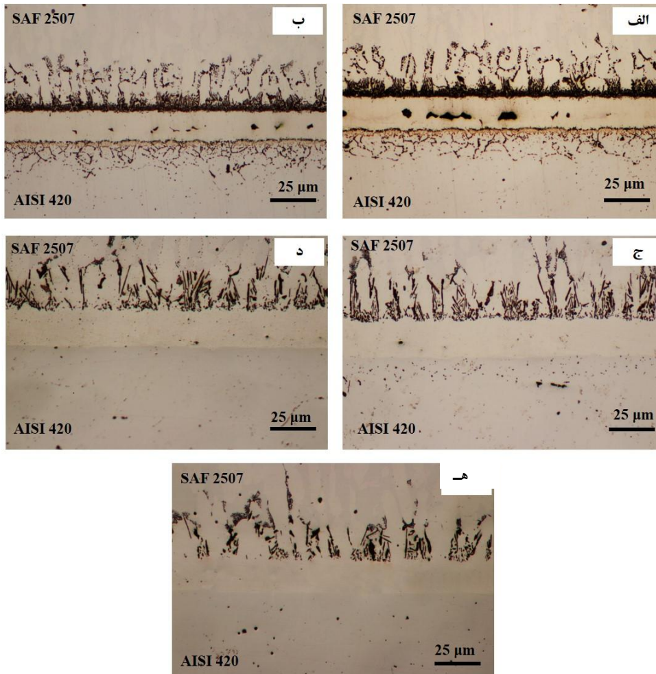
شکل ۸- تصاویر میکروسکوپی نوری از سطح مقطع اتصال نمونه‌های: الف) TH-1، ب) TH-15، ج) TH-30، د) TH-45 و ه) TH-60
