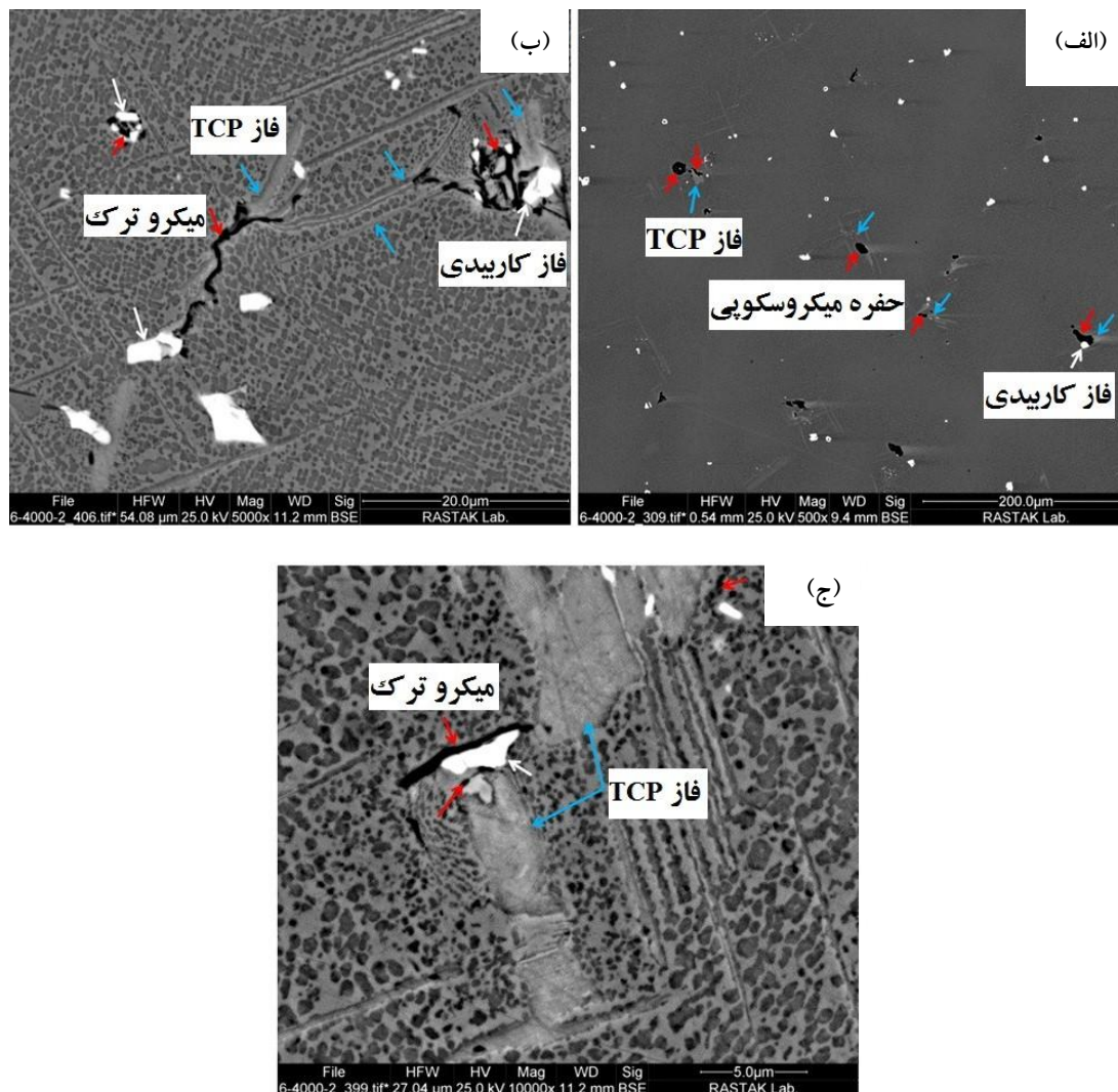
شکل ۹- تصاویر میکروسکوپی الکترونی روبشی از ریزساختار نمونه SXM4 پس از آزمون تنش گسیختگی نشان‌دهنده:
