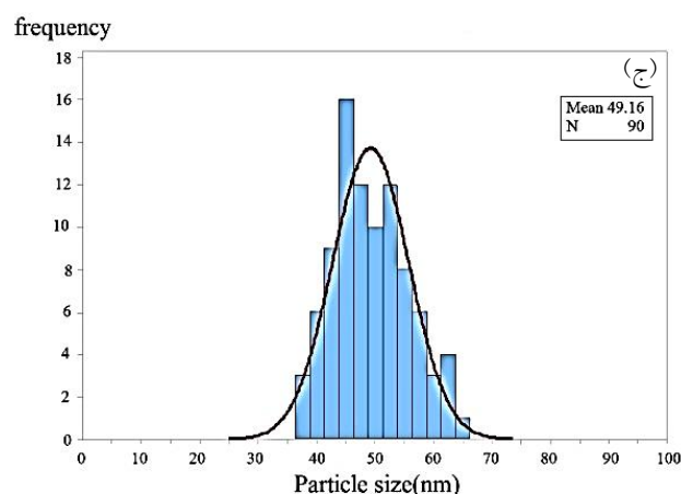
شکل ۱- تصاویر میکروسکوپی الکترونی روبشی گسیل میدانی ذرات فرآوری شده: (الف) در دمای 18^{\circ} درجه سانتی گراد به مدت ۶ ساعت، (ب) در دمای 13^{\circ} درجه سانتی گراد به مدت ۱۵ ساعت، (ج) نمودار توزیع اندازه ذرات در دمای 18^{\circ} درجه سانتی گراد به مدت ۶ ساعت و (د) نمودار توزیع اندازه ذرات در دمای 13^{\circ} درجه سانتی گراد به مدت ۱۵ ساعت
