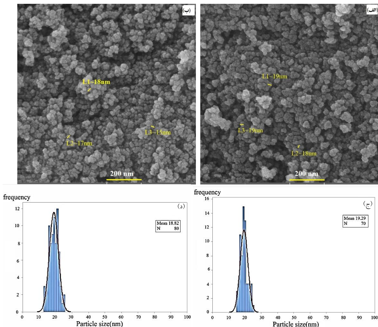
شکل ۲- تصاویر میکروسکوپی الکترونی روبشی گسیل میدانی نانوذرات فراوری شده: الف) در دمای ۱۴۰ درجه سانتی گراد به مدت ۱۵ ساعت، ب) در دمای ۱۵۰ درجه سانتی گراد به مدت ۱۵ ساعت، ج) نمودار توزیع اندازه ذرات در دمای ۱۴۰ درجه سانتی گراد به مدت ۱۵ ساعت و د) نمودار توزیع اندازه ذرات در دمای ۱۵۰ درجه سانتی گراد به مدت ۱۵ ساعت
