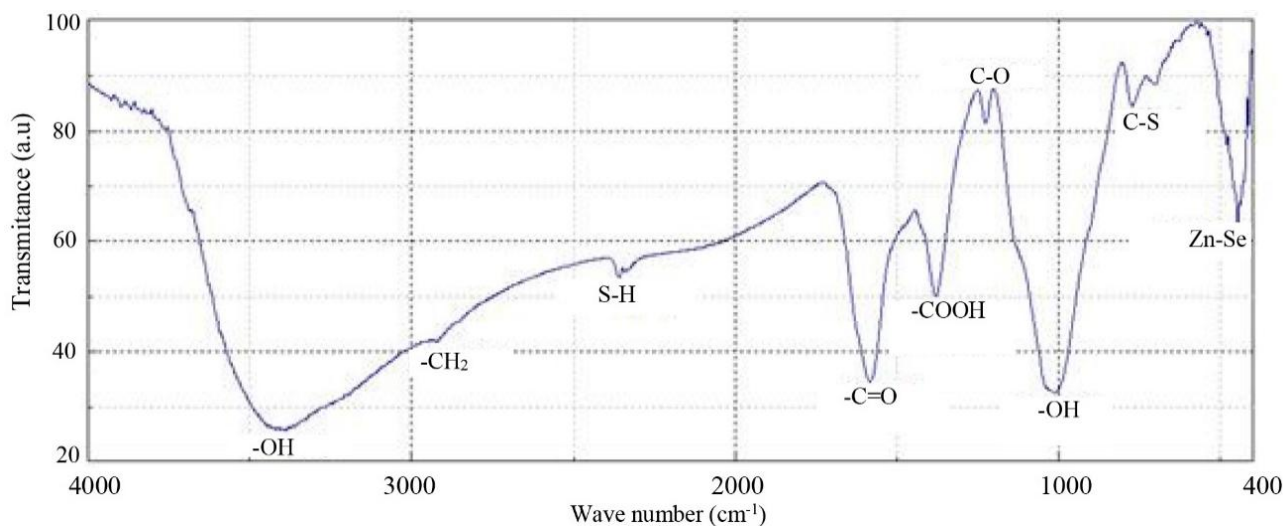
شکل ۱۲- طیف مادون قرمز تبدیل فوریه نانوذرات سلیند روی با عامل پوشاننده مرکپتو استیک اسید
