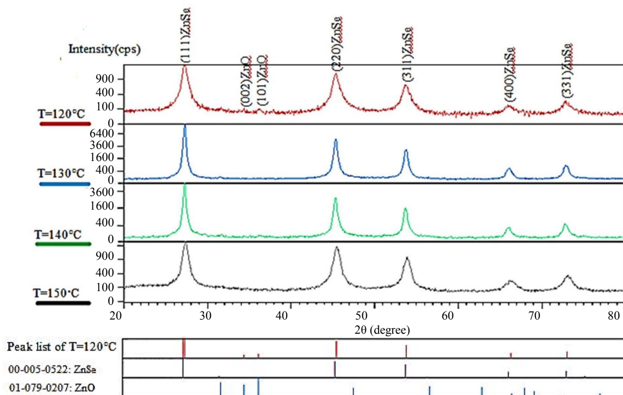
شکل ۶- الگوی پراش پرتو ایکس سلیند روی در دماهای مختلف سنتز در زمان ۱۵ ساعت
