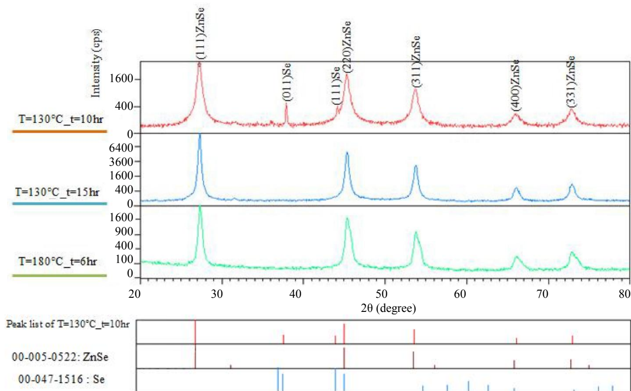
شکل ۷- الگوی پراش پرتو ایکس سلیند روی در زمانهای مختلف سنتز در دمای ۱۳۰ درجه سانتی گراد
