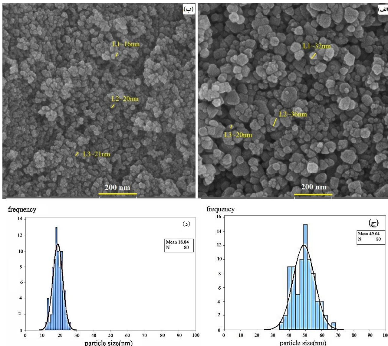
شکل ۳- تصاویر میکروسکوپی الکترونی روبشی گسیل میدانی نانوذرات با غلظت مرکپتو استیک اسید: الف) ۱/۰ میلی لیتر، ب) ۲/۰ میلی لیتر، ج) نمودار توزیع اندازه ذرات با غلظت مرکپتو استیک اسید ۱/۰ میلی لیتر و د) نمودار توزیع اندازه ذرات با غلظت مرکپتو استیک اسید ۲/۰ میلی لیتر
