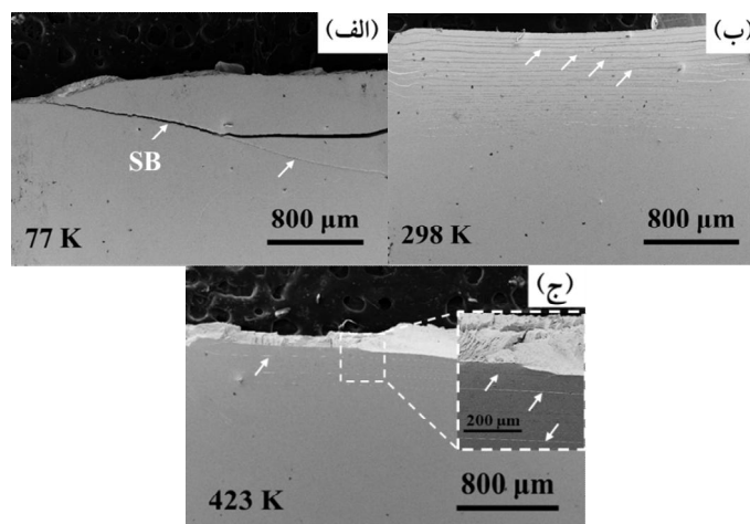
شکل ۷- تصاویر میکروسکوپی الکترونی روبشی نشر میدانی از سطح کشتی نمونه‌های خمش مربوط به آلیاژ خم شده در دماهای: (الف) ۷۷، (ب) ۲۹۸ و (ج) ۴۲۳ کلوین و نرخ خمش ۰/۲ میلی‌متر بر دقیقه (پیکان‌ها نوارهای برشی را نشان می‌دهند).
