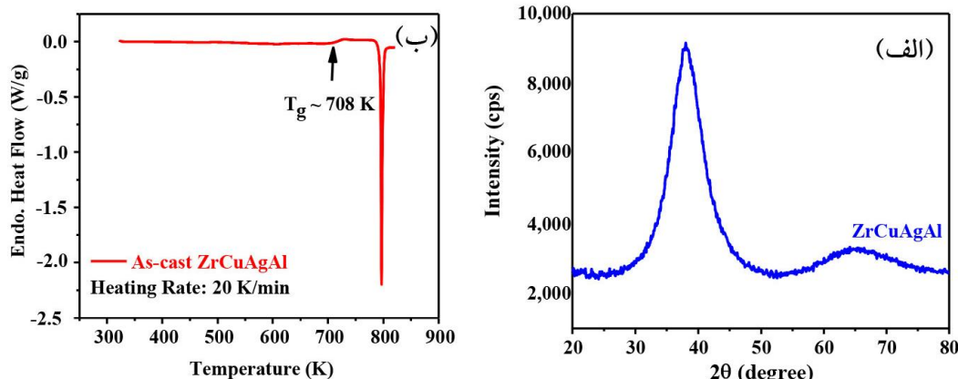
شکل ۱- الف) الگوی پراش پرتو ایکس (XRD) و ب) نمودار آزمون گرماسنجی روبشی تفاضلی
