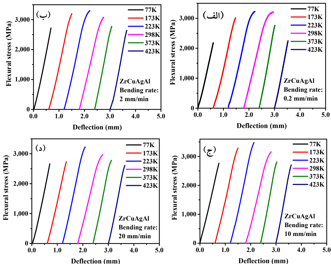
شکل ۲- منحنی‌های تنش - جابه‌جایی خمشی آلیاژ Zr_{46}(Cu_{4.5/5.5}Ag_{1/5.5})_{46}Al_8 خم شده در دماهای مختلف و با نرخ‌های خمش:
