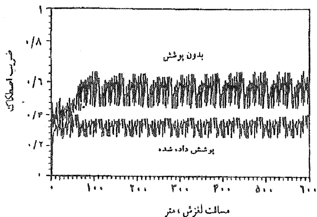
شکل ۹- نمودار ضریب اصطکاک بر حسب مسافت لغزش برای نمونه فولادی بدون پوشش و نمونه ای با پوشش بهینه از ترکیبات بین فلزی Fe-Al (بارگذاری به صورت مرحله ای با نرخ 30\text{ N}/1000\text{ m} )
