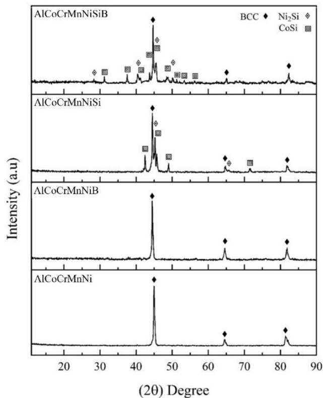
شکل ۴- الگوهای پراش پرتو ایکس پودر آلیاژهای \text{AlCoCrMnNiX} ( X = \text{B, Si} ) پس از عملیات آنیل در دمای 900^\circ\text{C} درجه سانتی‌گراد به مدت 10 ساعت
