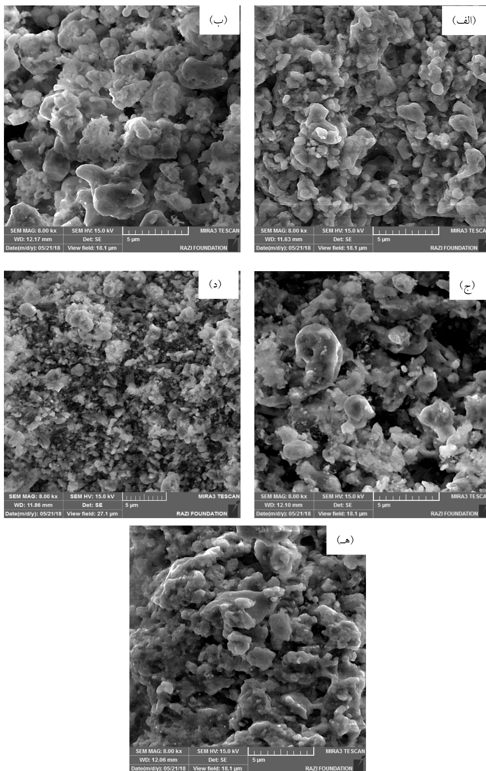
شکل ۶- تصاویر میکروسکوپی الکترونی روبشی ذرات پودری آلیاژهای: الف) \text{AlCoCrMnNi} ، ب) \text{AlCoCrMnNiB} ، ج) \text{AlCoCrMnNiSi} و د) \text{AlCoCrMnNiSiB} پس از انجام عملیات آنیل در دمای 900^\circ\text{C} درجه سانتی‌گراد به مدت ۱۰ ساعت و ه) آلیاژ \text{AlCoCrMnNi} پس از انجام عملیات آنیل در دمای 900^\circ\text{C} درجه سانتی‌گراد به مدت ۱۵ ساعت
