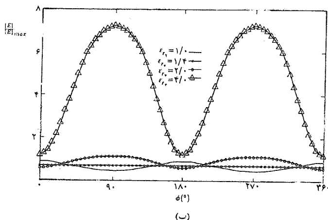
شکل ۱۰- تأثیر ثابت عایقی روبنا بر روی نماد تشعشی آنتن مثال (۶)، f=9\text{GHz}
