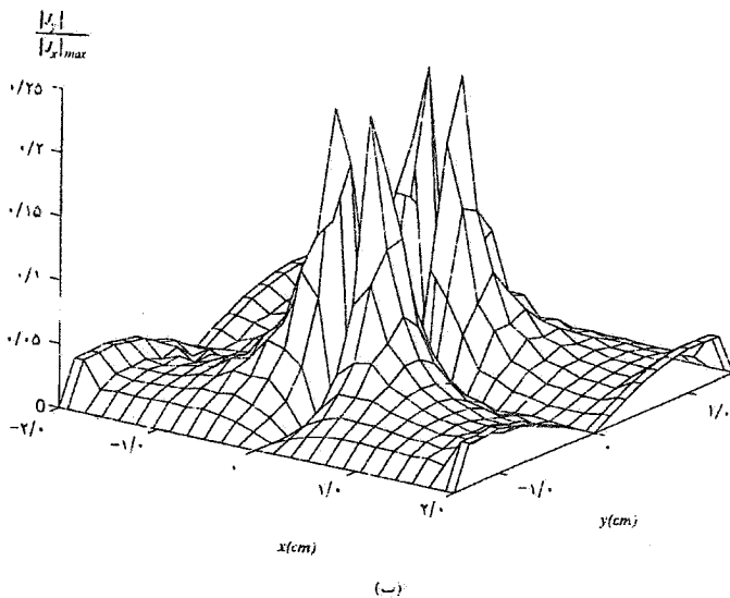
شکل ۵- توزیع جریان روی آنتن، l_a = 1/1 , b = 3 \text{ cm} , a = 4 \text{ cm} , x_p = y_p = 0 , l_s = 1/2 \text{ cm} , w_f = 0.44 \text{ cm} , w_a = 0.16 \text{ cm} مستقارن، f = 2.23 \text{ GHz} و d_1 = d_f = 0.16 \text{ cm} , \epsilon_{rf} = \epsilon_{ff} = 2/54 (الف) - مؤلفه E_x (ب) - مؤلفه E_y
