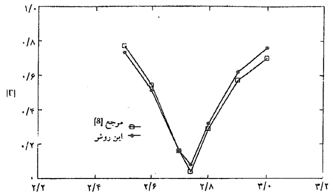
شکل ۴- تغییرات ضریب انعکاس آنتن شکافی مثال (۱) برحسب فرکانس ابعاد شکاف w_f = 0.635 \text{ cm} , 4/0 \text{ cm} \times 0.1016 \text{ cm} , d_f = 0.203 \text{ cm} , \epsilon_{rf} = 2/2 , l_s = 0.22 \text{ cm}
