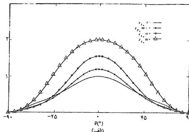
شکل ۱۰- تأثیر ثابت عایقی روبنا بر روی نماد تشعشی آنتن مثال (۶)، f=9\text{GHz}
