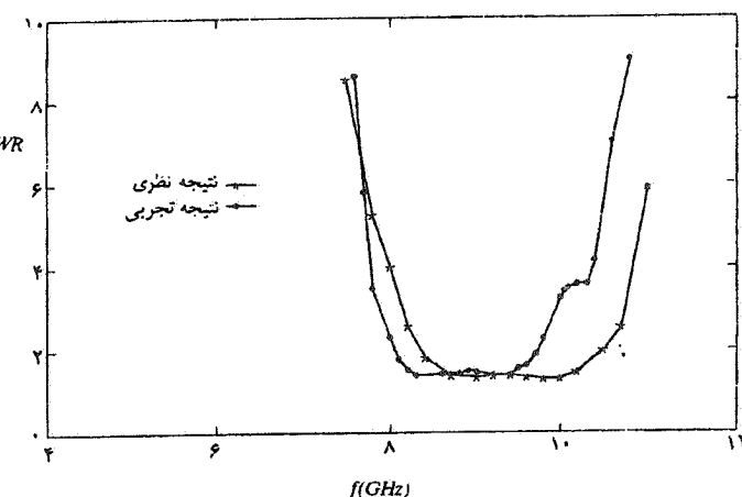
شکل ۷- نتیجه تجربی و نظری برای VSWR آنتن مثال (۴)، w_a=0.4\text{cm} ، d_a=0.75\text{cm} ، b=1/1\text{cm} ، a=0.7\text{cm} ، d_1=0.317\text{cm} ، \epsilon_{rf}=6/15 ، w_f=0.9\text{cm} ، d_s=0.11\text{cm} ، d_f=0.614\text{cm}
