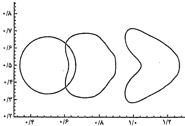
شکل ۶- تغییر شکل قطره در Re_l=200 و Re_g=20
