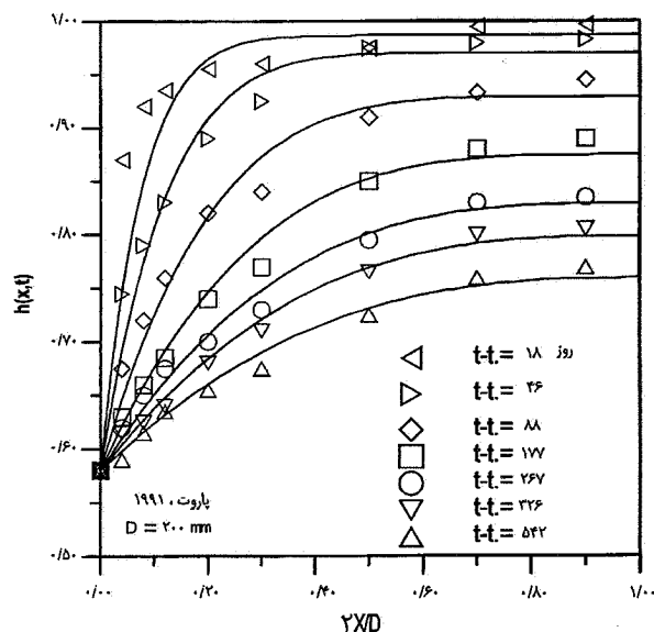
شکل ۴- پروفیل توزیع رطوبت نسبی در مقطع دال آزمایش پاروت [۱۰] برای عمرهای مختلف
