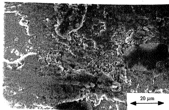
شکل ۶- توپوگرافی SEM سطح سایش عضو مقابل فولادی
