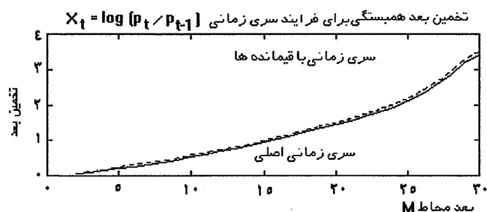
شکل (۴): بعد همبستگی سری اصلی و سری مانده ها به ازای مقادیر متناظر M
