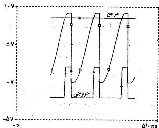
ج - سیگنالهای ورودی و خروجی مقایسه کننده
