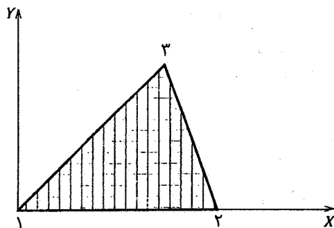
شکل ۱- صفحه مثلثی ارتوتروپیک
