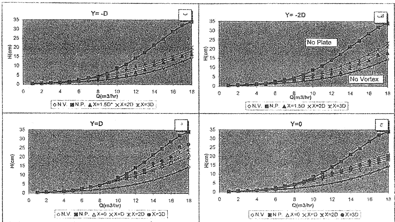
شکل ۶- نمونه‌هایی از نتایج تأثیر فواصل مختلف X در عمقهای آزمایش شده برای صفحه‌ای به ابعاد A=1.5D \times 2D و قطر خروجی 7.5 cm (بدون گرداب = N.V., بدون صفحه = N.P.)
