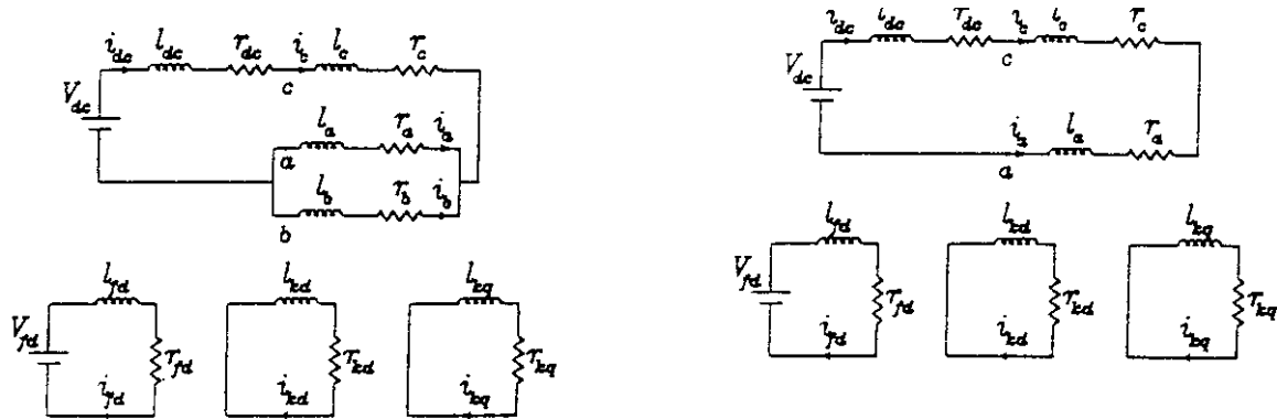
شکل ۲- شمای الکتریکی حالت کاری بین دو کموتاسیون
