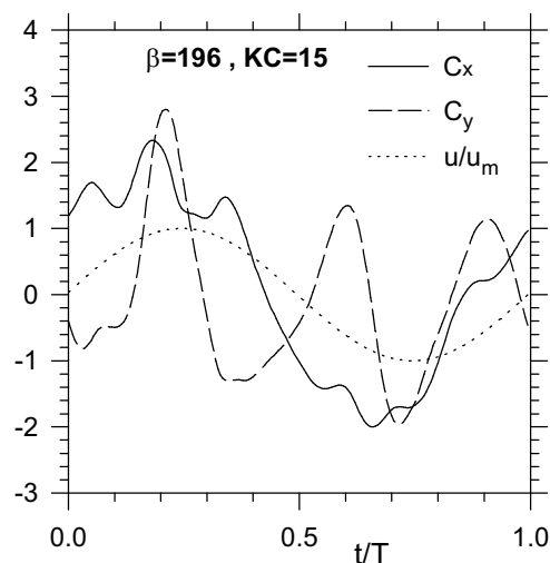
شکل ۸- تغییرات ضرایب نیرو در یک سیکل
