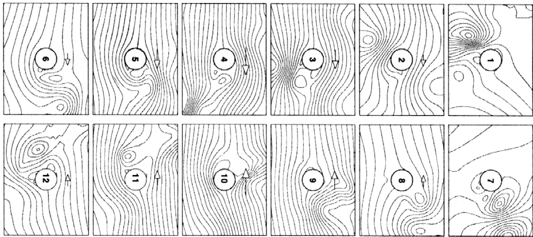
شکل ۷- از راست به چپ به ترتیب خطوط وردنیستی و خطوط جریان برای حالت‌های استوانه نوسانی و جریان نوسانی به ازای \beta = 196 , KC = 15.0
