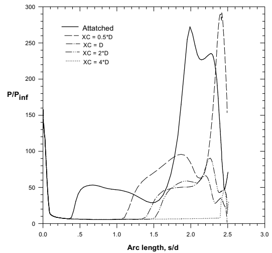
شکل ۸- توزیع فشار بر روی سطح سرجنگی برای حالت متصل و فواصل مختلف سر و بدنه شکل ۹- ضریب نیروی مقاوم روی سرجنگی در فواصل مختلف سر و بدنه
