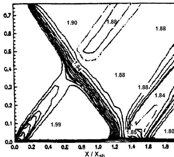
شکل ۱۳- خطوط ثابت ماخ برای جریان با M=2
