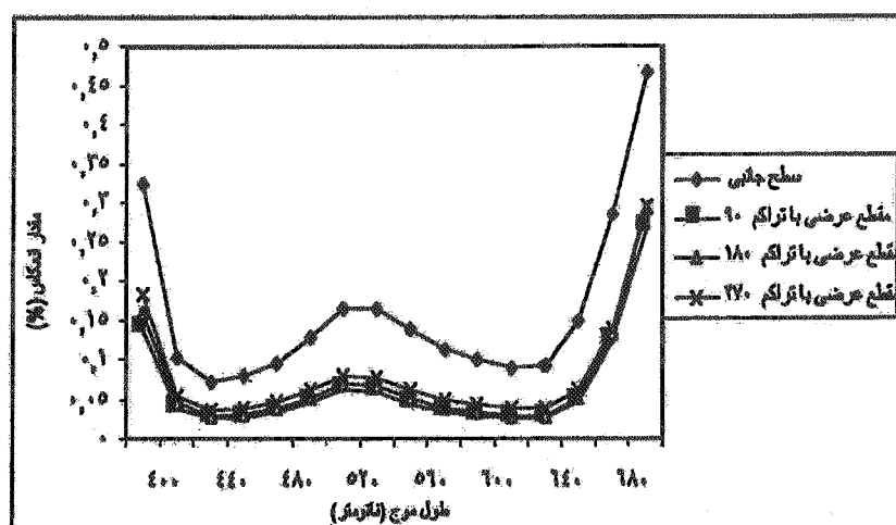
شکل ۱۰ - منحنی انعکاس طیفی نمونه شماره ۶ در امتداد طولی و مقطع عرضی با تراکمه های مختلف
