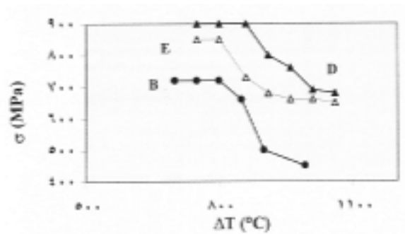
شکل ۱۴- تغییرات استحکام شکست نمونه‌های B و D و E نسبت به \Delta T برای سیکل‌های شوک گرمایی مختلف
