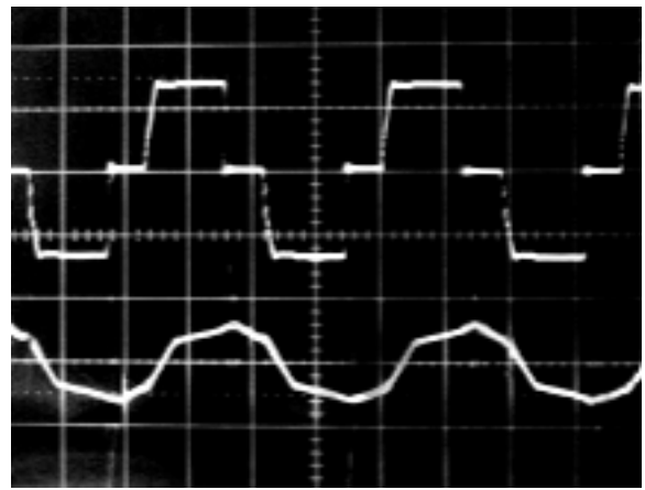
شکل ۱۳- ولتاژ و جریان اولیه ترانس (با ضریب وظیفه زیاد)
