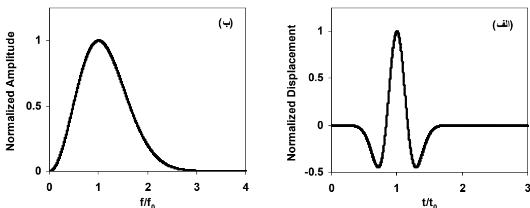
شکل ۲ - الف- تاریخچه زمانی و ب- طیف دامنه فوریه موج ریکر
