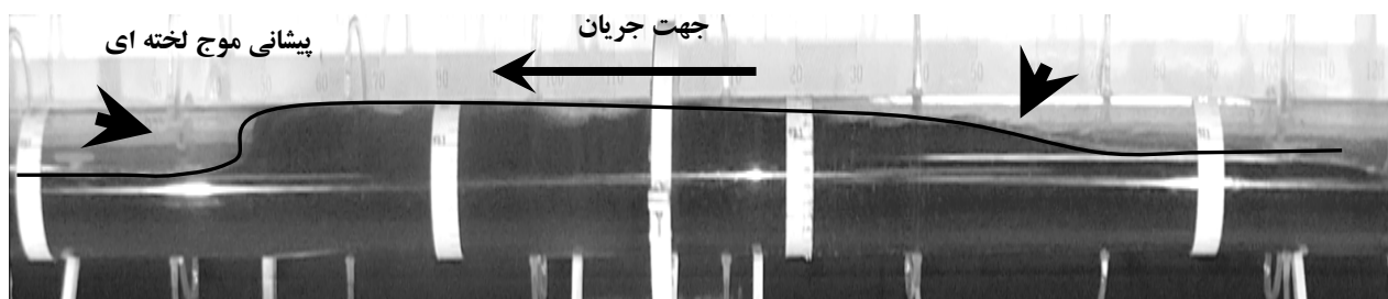
شکل ۶- نمونه‌ای از لخته تشکیل شده در مجرا
