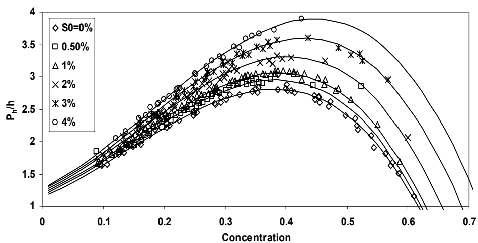
شکل ۱۲- تغییرات P_h/h بر حسب غلظت متوسط در شبیه‌های مختلف
