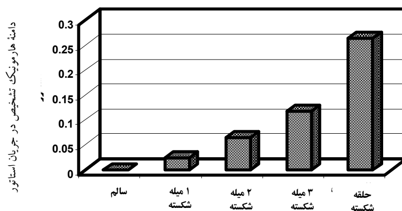
شکل ۵- مقایسه دایمۀ هارمونیک f_s(1+2s) برای انواع حالات رتور و گشتاور بار مشابه
