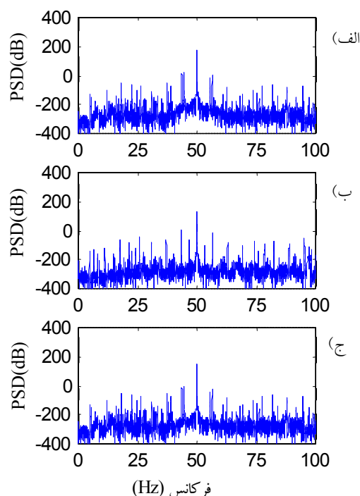
شکل ۹- نتایج طیف فرکانسی موتور آزمایشگاهی در فاصله 0-100 Hz الف) رتور سالم ب) رتور با حلقه انتهایی برش زده شده ج) رتور با دو میله برش زده شده
