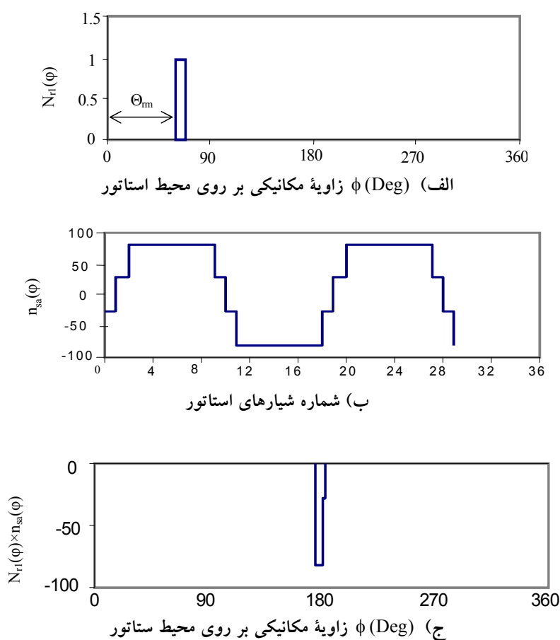
شکل ۱- فاصله مراحل مربوط به محاسبه اندوکتانس L_{ar1} :
