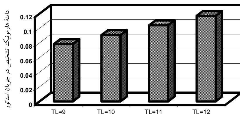
شکل ۶- مقایسه دانه هارمونیک f_s(1+2s) در حالت سه میله شکسته و گشتاورهای بار مختلف
