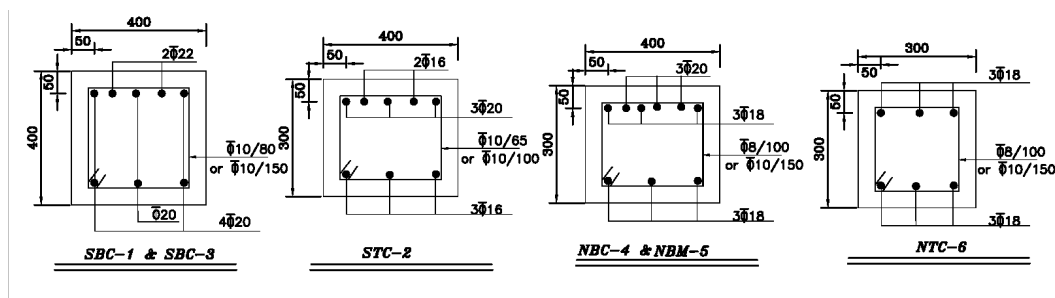
شکل ۱- مشخصات مقطع و فولادگذاری اعضا در زیر سازه اصلی (واحدها به mm است)
