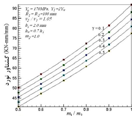
شکل ۱۱- تغییرات گشتاور نورد بر اساس نسبت‌های مختلف از دو لایه ورق
